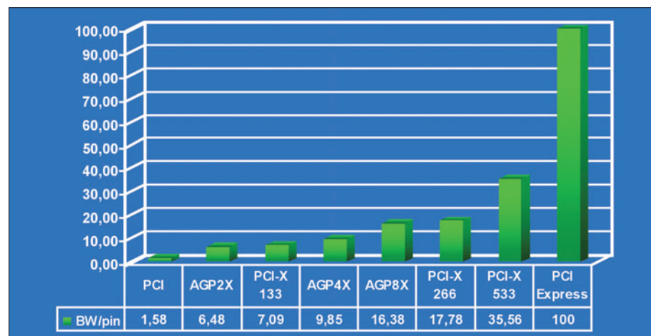
Figure 2 : Rapport de capacité de transport par contact pour différentes interfaces.
